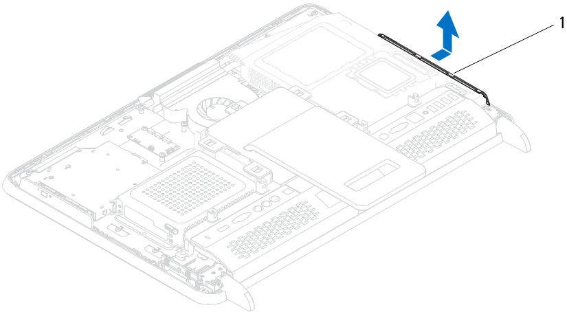
1 I/O-zijpaneel
