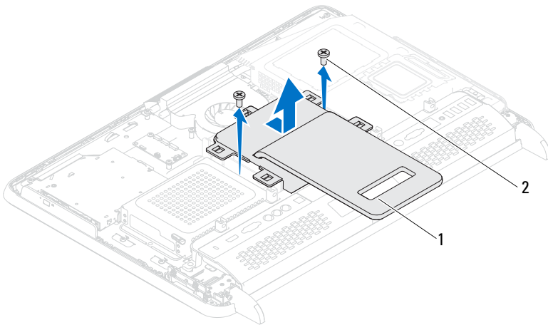
1 beeldschermconstructie 2 schroeven (2)
