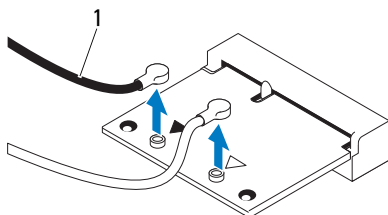
1 antennekabels (2)
